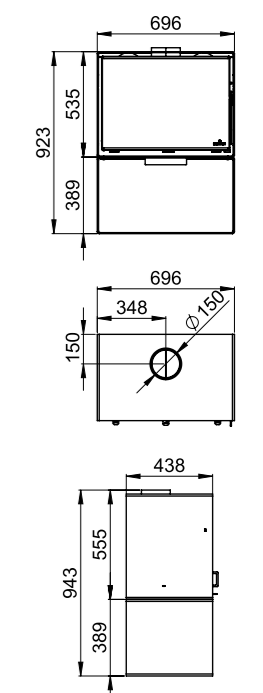
CAIRO-70-BOX +KIT-VER-70BOX (Kit Vermiculita) + L-70BOX (Leñero - Woodshed - Lenheiro) CAIRO-70-BOX +KIT-FIR-70BOX (Kit Firetek) + L-70BOX (Leñero - Woodshed - Lenheiro)
